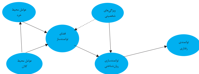
شکل ۳: برازش کلی مدل
