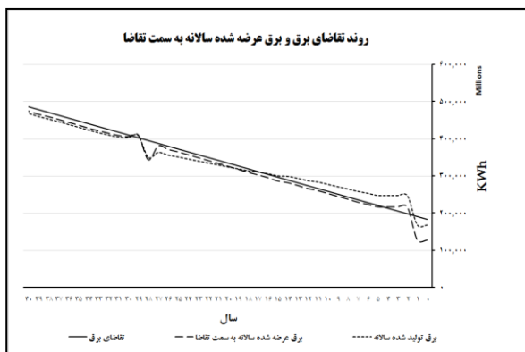
نمودار ۲: روند تغییرات تقاضای سالانه برق، تولید سالانه الکتریسیته و انرژی الکتریکی عرضه شده به بخش تقاضا
